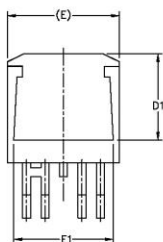
VIEW A-A
