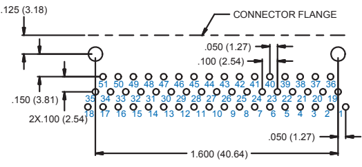
51 PIN M83513/17-G
